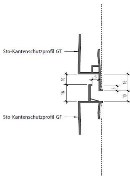
Utförande StoProfile Edge GT/GF
