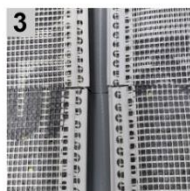
Fogutformning med Sto Fogprofil E
